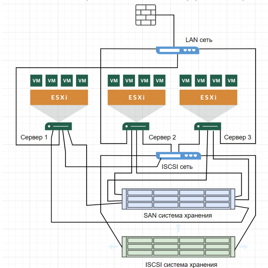
Логическая схема реализации подсистемы виртуализации – рис. 1
